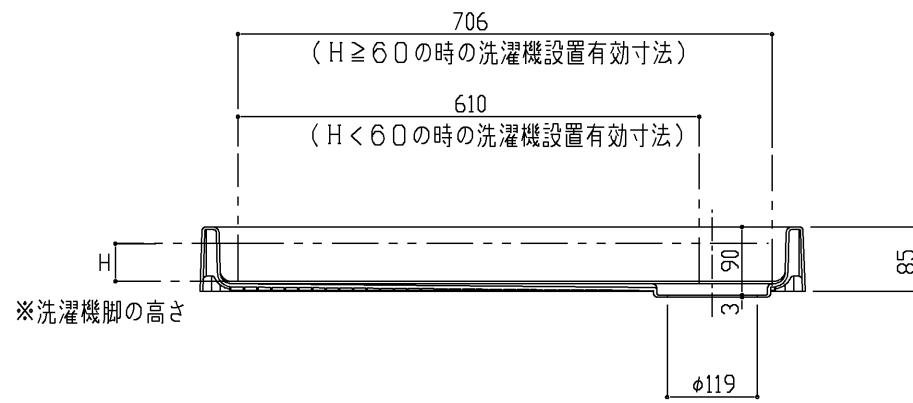
断面A-A
